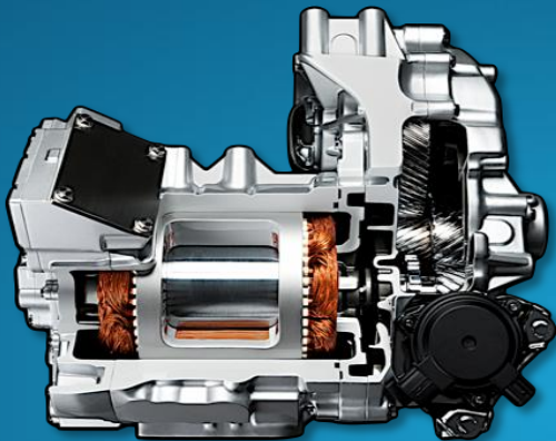
Powertrain 80KW
